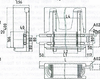
Рис. 2 Конвектор «Универсал С» проходной, правого исполнения с модулем «А02»
